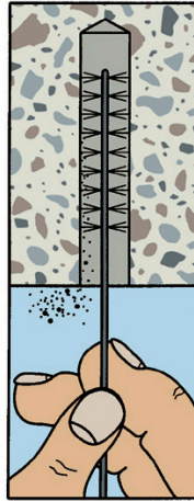
Borehullsrengjøring: Blåse - børste
