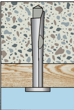
Innhamret stålstift sikrer forankring
